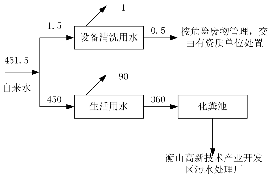
图 2-1 水平衡图 \text{m}^3/\text{a}
